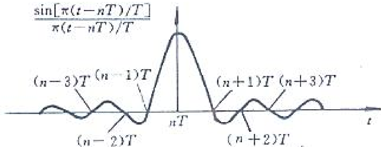
图 2—8 内插函数
