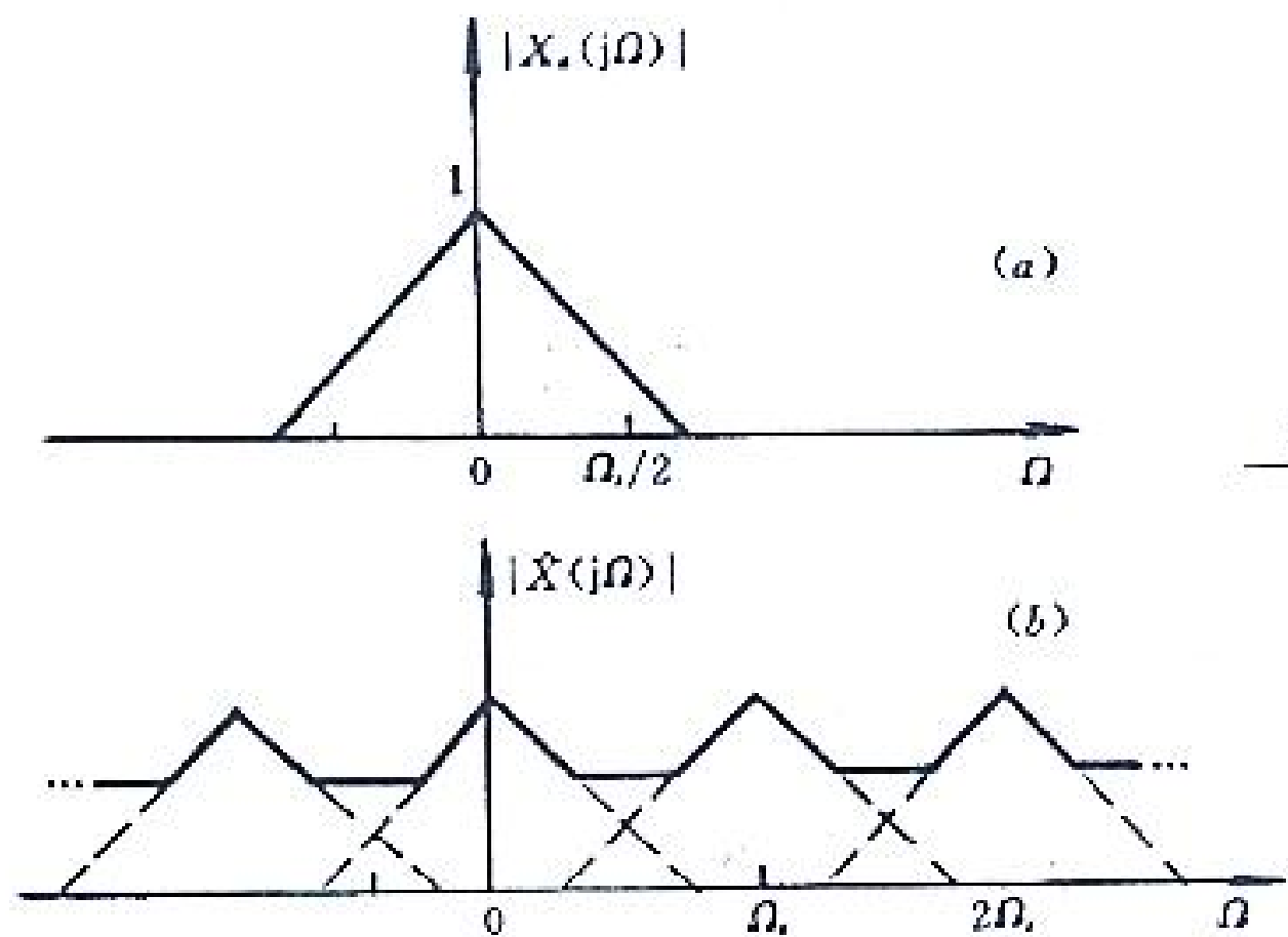
图 2-4 频谱的混叠
